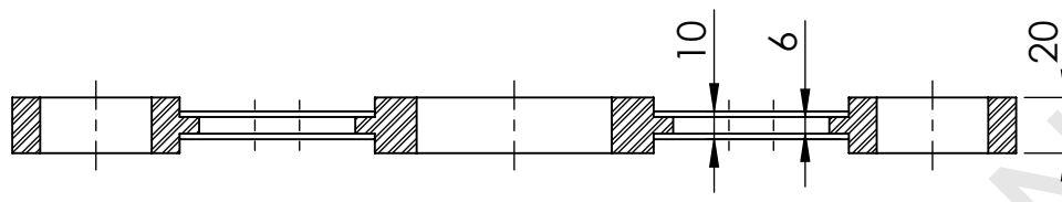
SECCIÓN A-A
