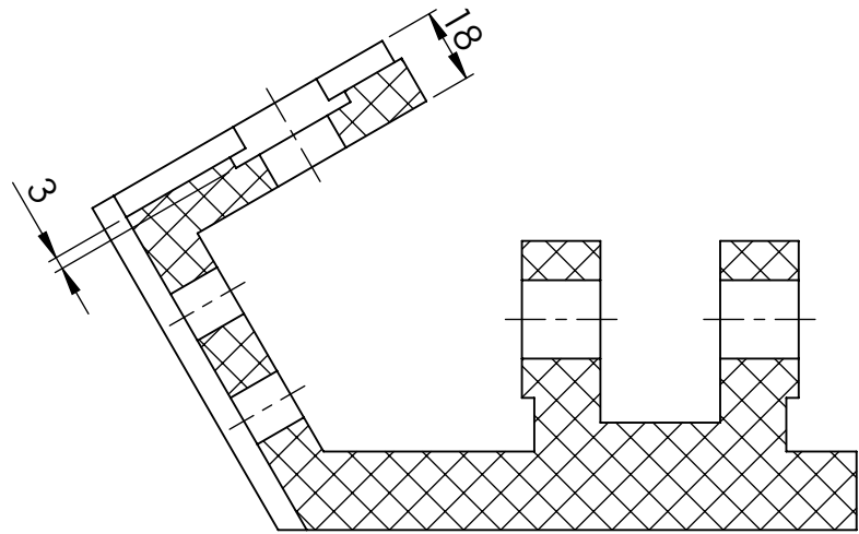
SECCIÓN C-C
