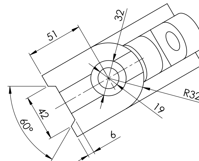
VISTA A
