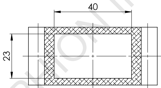
SECCIÓN A-A
