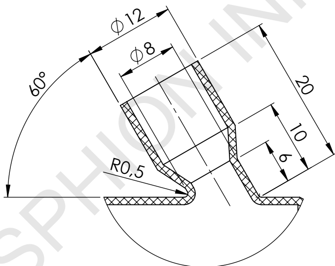
DETALLE Y 2 : 1
