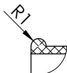
DETALLE X 2 : 1
