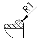
DETALLE Z 2 : 1
