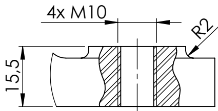
DETALLE Z 1 : 1
