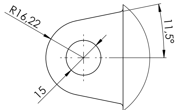
DETALLE Y 1:1
