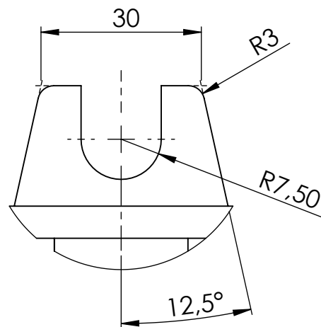
DETALLE Z 1:1
