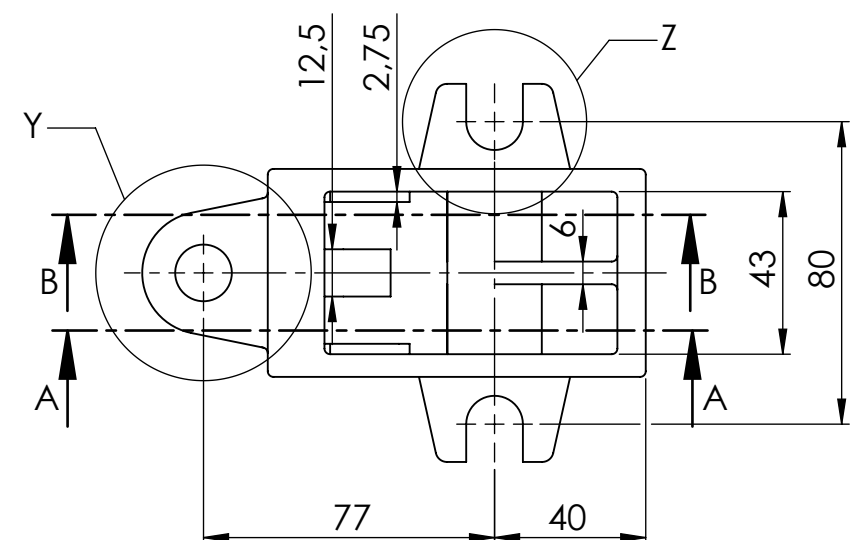
SECCIÓN A-A
