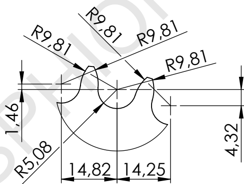
DETALLE Z 1 : 1
