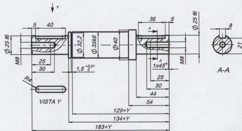
EIXO AÇO 1050
