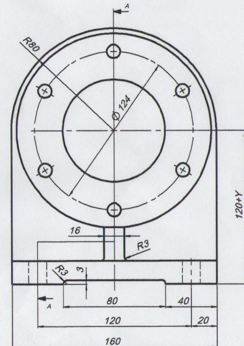
SUPOORTE AÇO 1020
