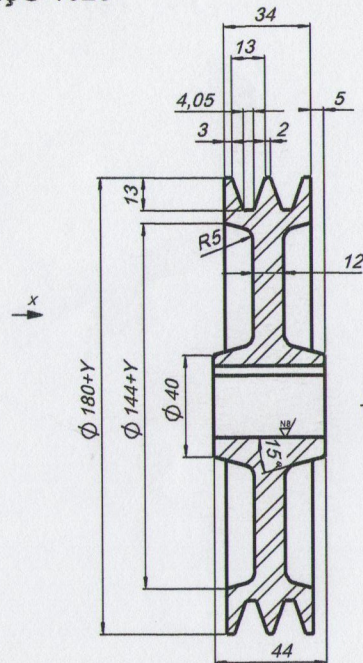
POLIA MOVIDA AÇO 1020
