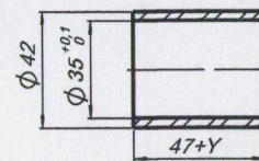
BUCHA DISTANCIADORA AÇO 1020
