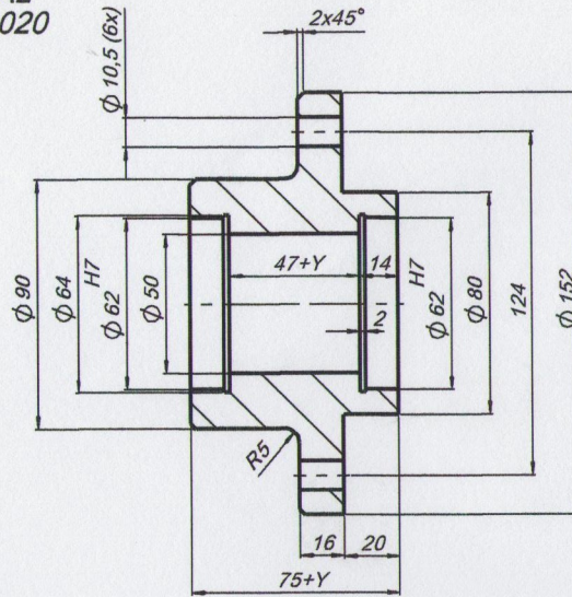
BUCHA DISTANCIADORA AÇO 1020
