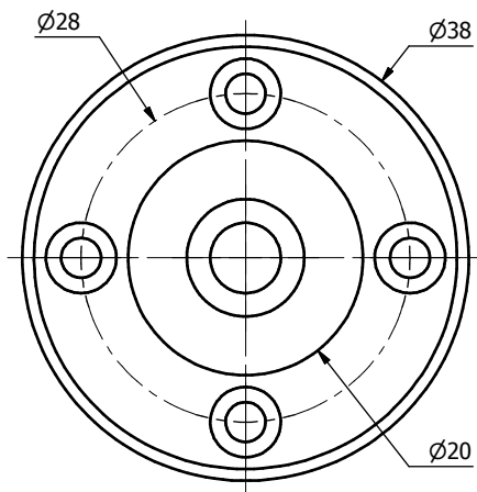
St.12.00 (Culata Cilindro Principal)
