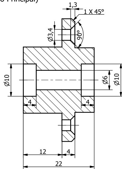
St.12.00 (Culata Cilindro Principal)
