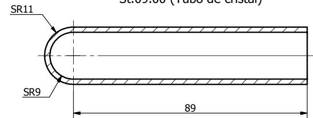
St.09.00 (Tubo de cristal)
